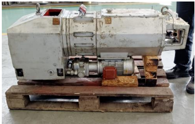
维修ZSE 50齿轮箱 Repair ZSE 50 gearbox
